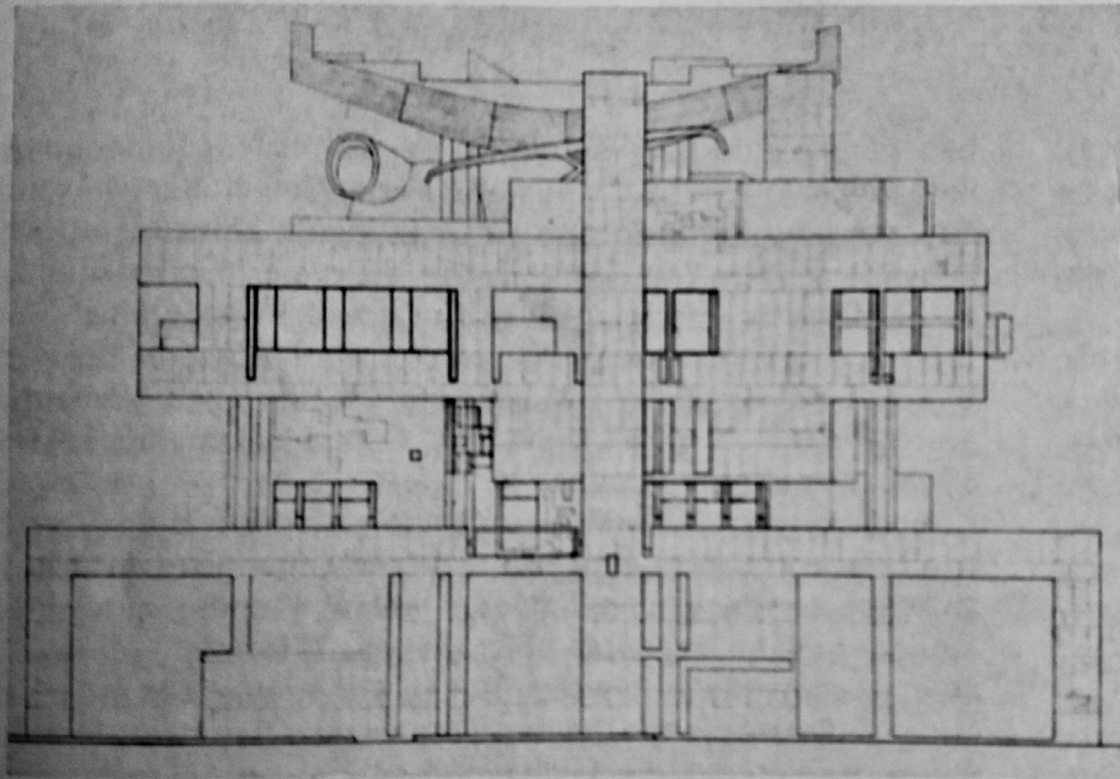
Elévation de la façade nord-ouest
