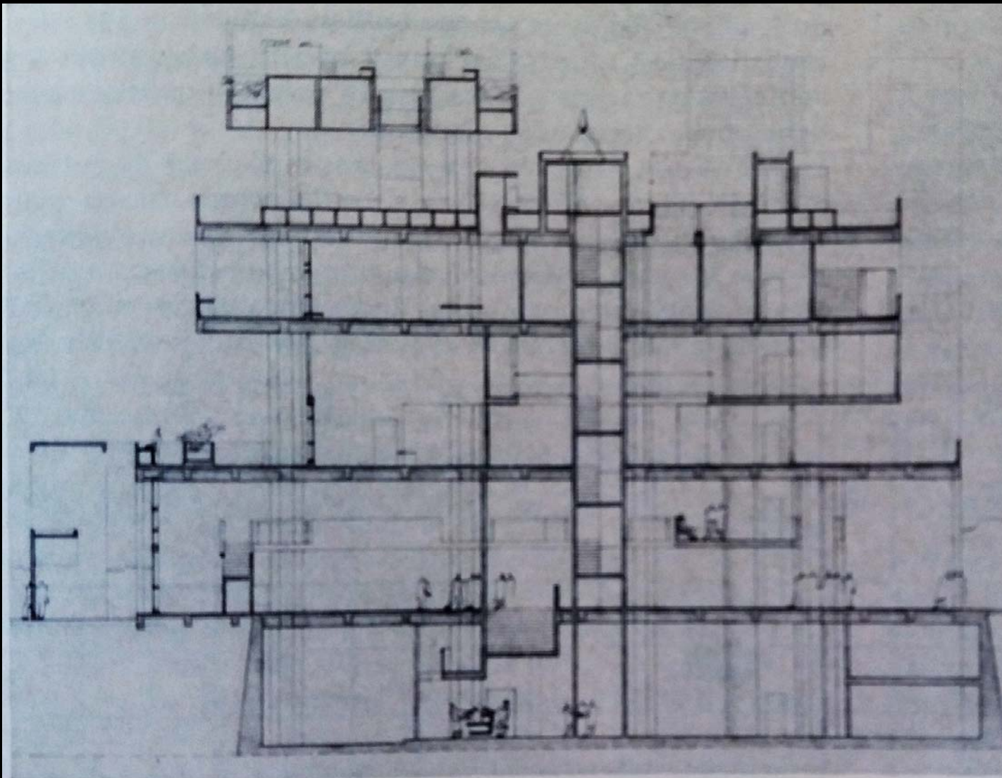
Coupe nord-ouest/sud-est
